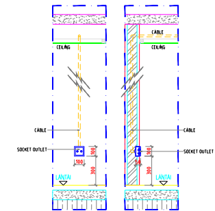
08 DETAIL PERANGKAT
